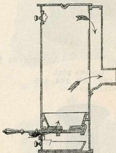
Coupe verticale du foyer du Calorifère " Revinois "
